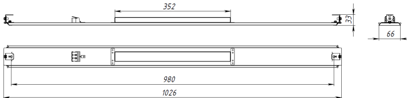
Рисунок 4 - Габаритные размеры при комплектации с уголком для накладного монтажа (на примере Liner Basic 1026x66x25).
